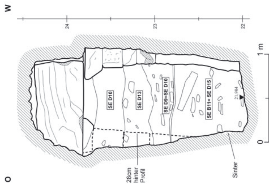
Abb. 327: ES1, Aristion-Leitung, S 1/2006, Schnitt
