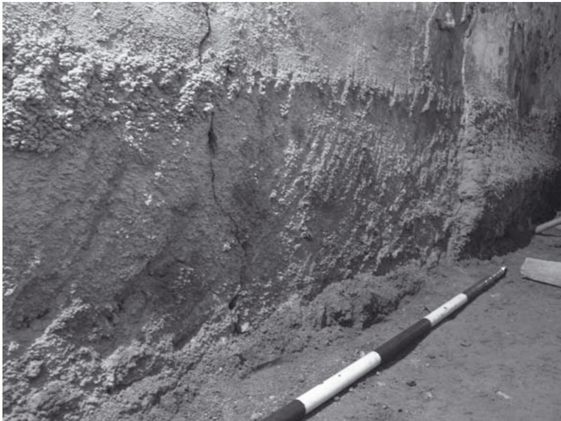
Abb. 318: ES1, Aristion-Leitung, Sinterablagerungen an der östlichen Leitungswandung
