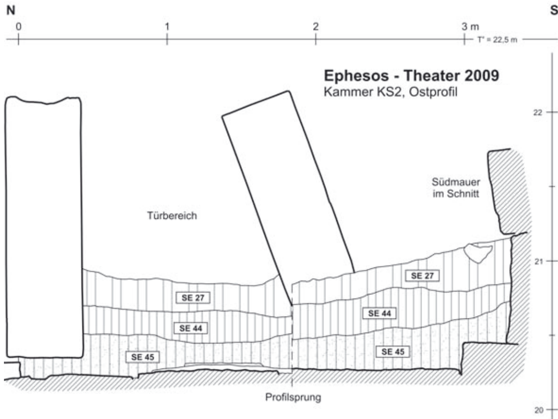
Abb. 366: Kammer KS2, O-Profil
