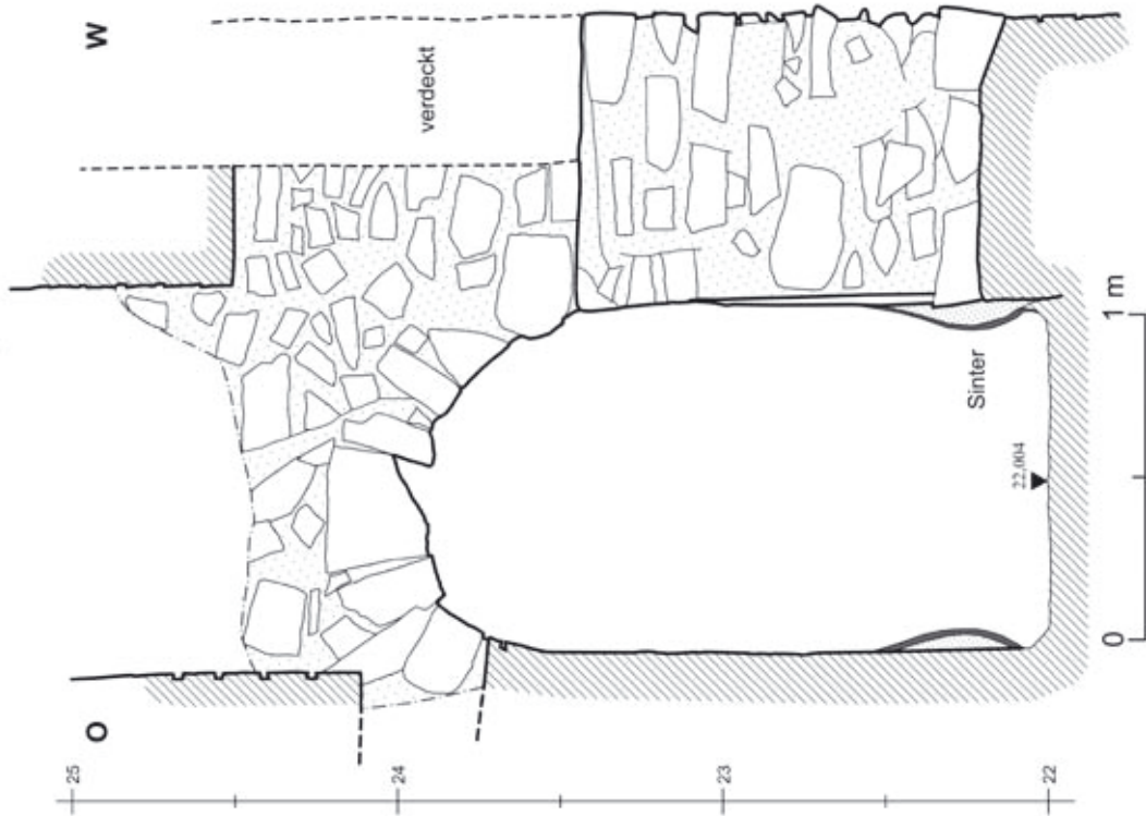
Ephesos - Theater 2006 Ost-Westschnitt durch Wasserleitungskanal bei lfm. 0
