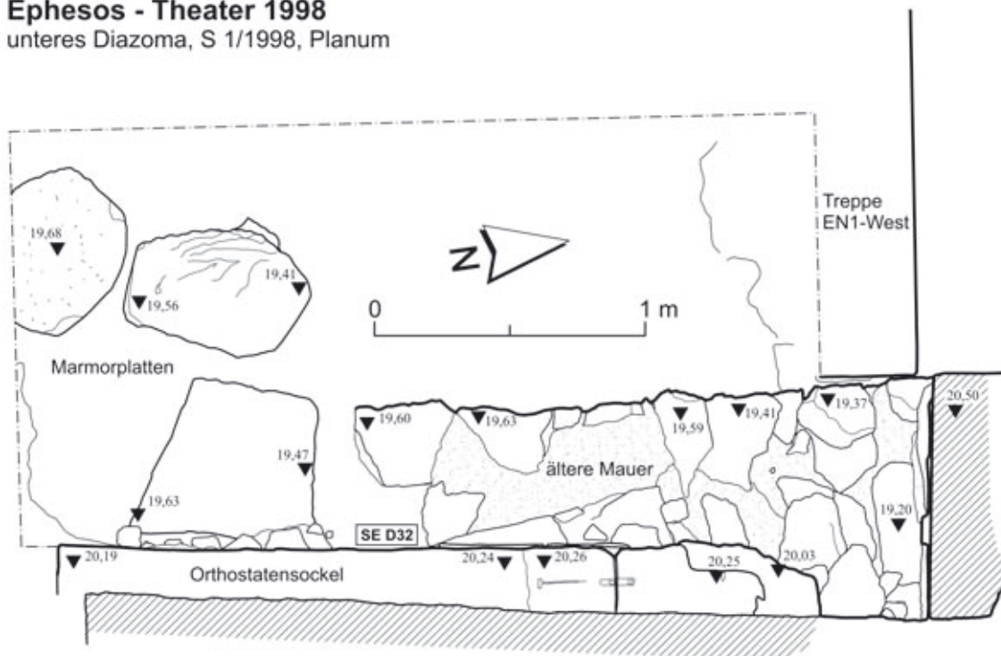
Abb. 281: Nördlicher Treppenaufgang, S 1/98, Fundamentierung (1. Phase), Planum
